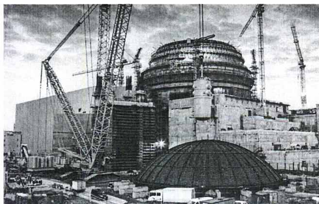
Монтаж корпуса реактора ЛАЭС-2 методом «Open-Top»
